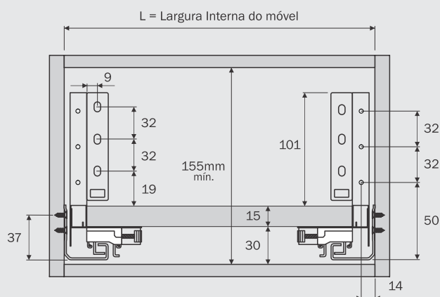
Corte dos painéis (15mm)
